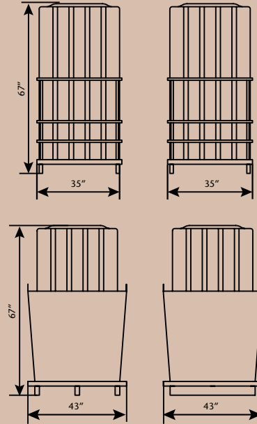
Dimensions
